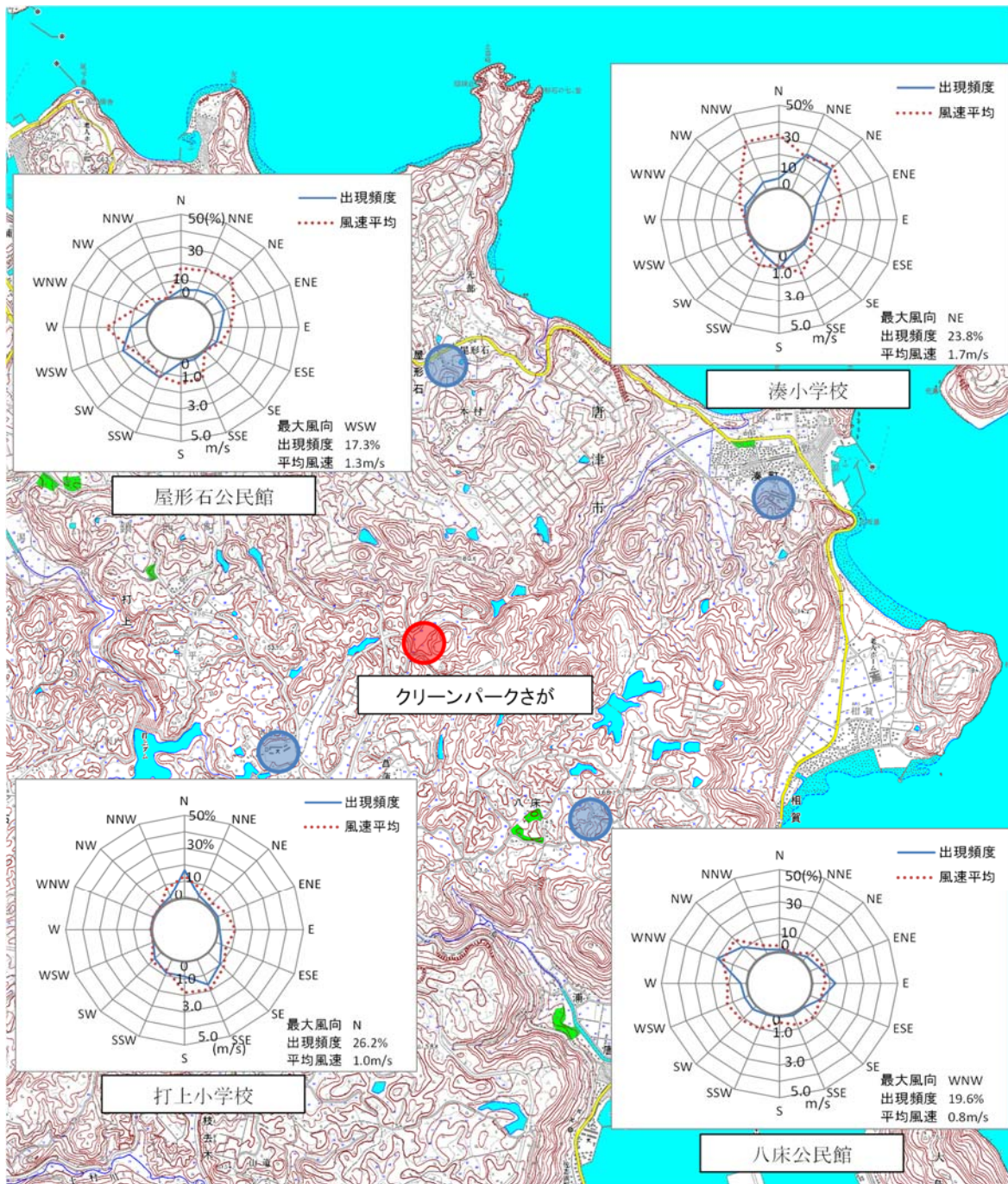
図 3-2-5 風配図
